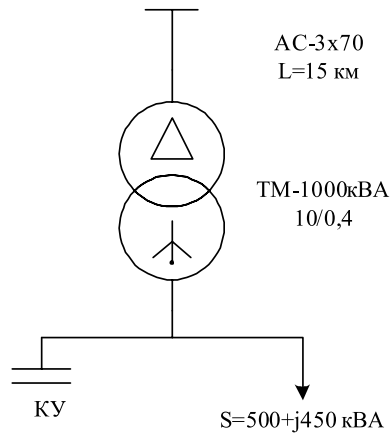
Рисунок 2 – Розрахункова схема
