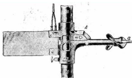
Рисунок 6 Вертушка Отта-IV
