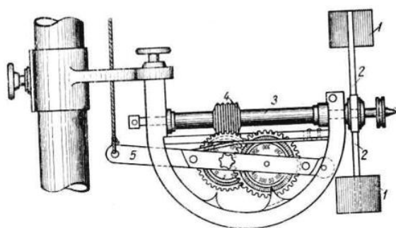
Рисунок 1 Механический счетчик Рейнгарда Вольмана
