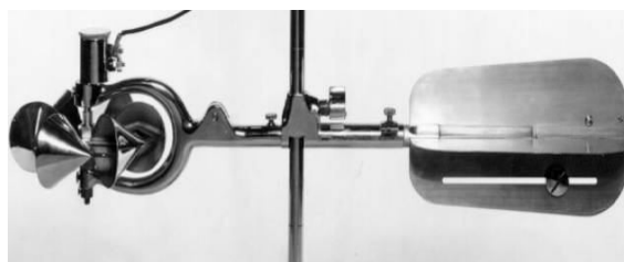
Рисунок 4 Вертушка Прайса USGS TYPE AA MODEL 6200 (Rickly Hydrological Company, США)
