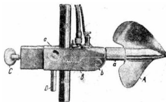
Рисунок 7 Вертушка Отта-V
