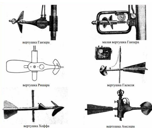
Рисунок 8 Вертушки конца XIX в.
