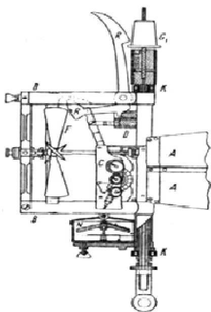
Рисунок 2 Механическая вертушка Экмана — Мерца
