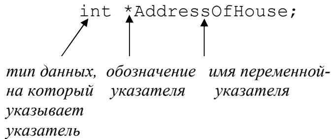
Рисунок 2.1 — Объявление переменной-указателя
